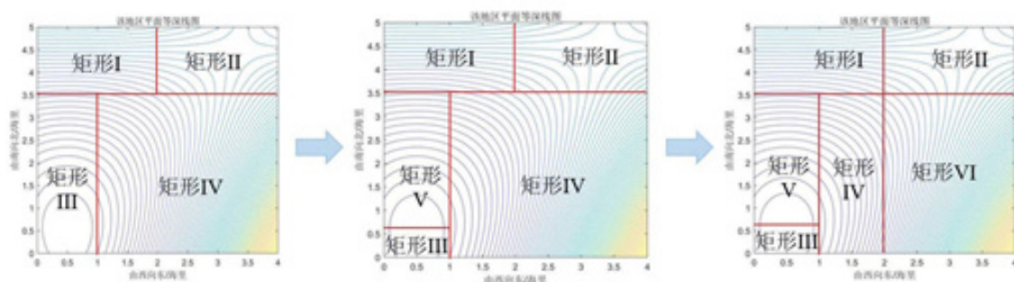
图 25: 海域逐步划分过程
