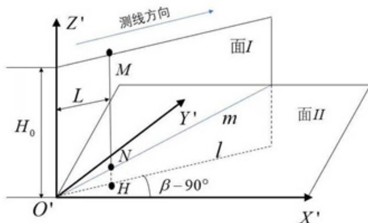
图 12: 海水深度计算
